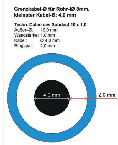
Bild 267 links: oberer Grenzkabel-Ø für SD-Innen-Ø 8,0 mm Bild 268 rechts: unterer Grenzkabel-Ø für SD-Innen-Ø 8,0 mm
